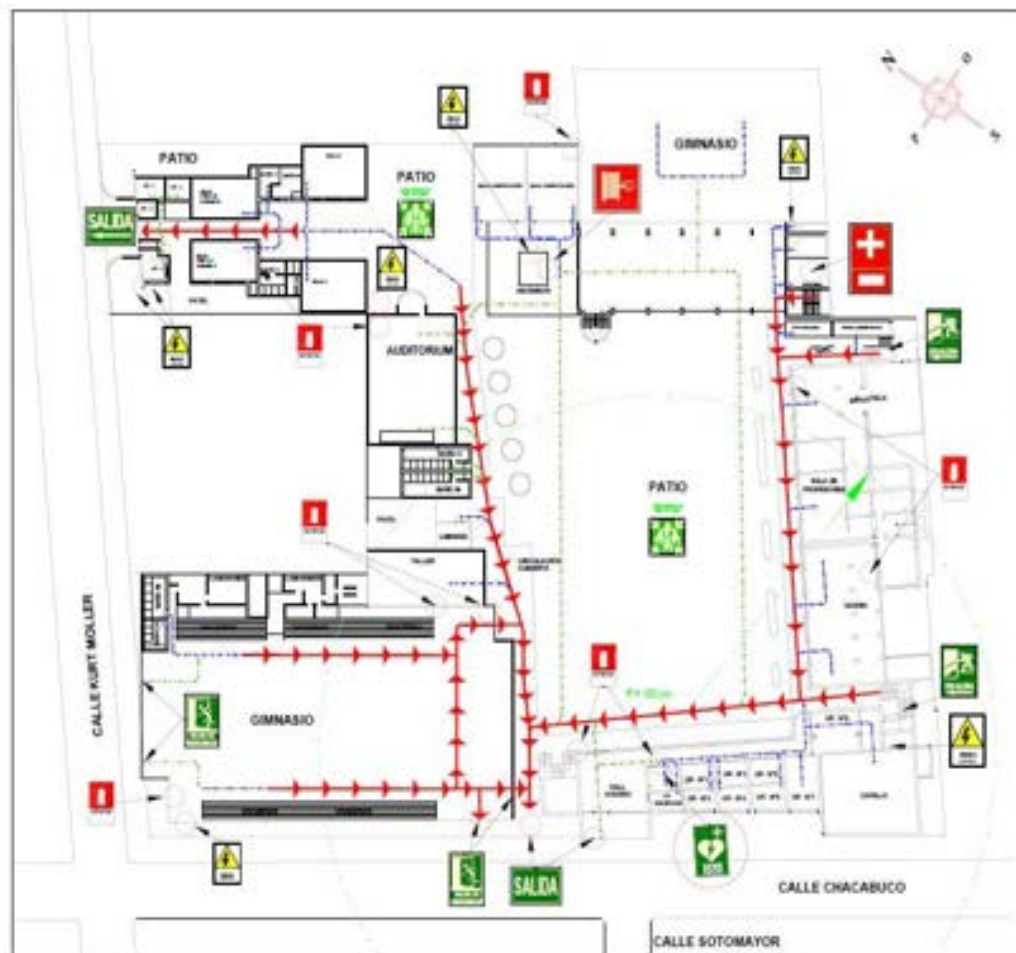
PLANTA 1º NIVEL, INSTITUTO LINARES, PLANO GENERAL DE DISTRIBUCIÓN SEÑALIZACIÓN VÍAS DE EMERGENCIA Y DEA. Escala: 1:250.-
