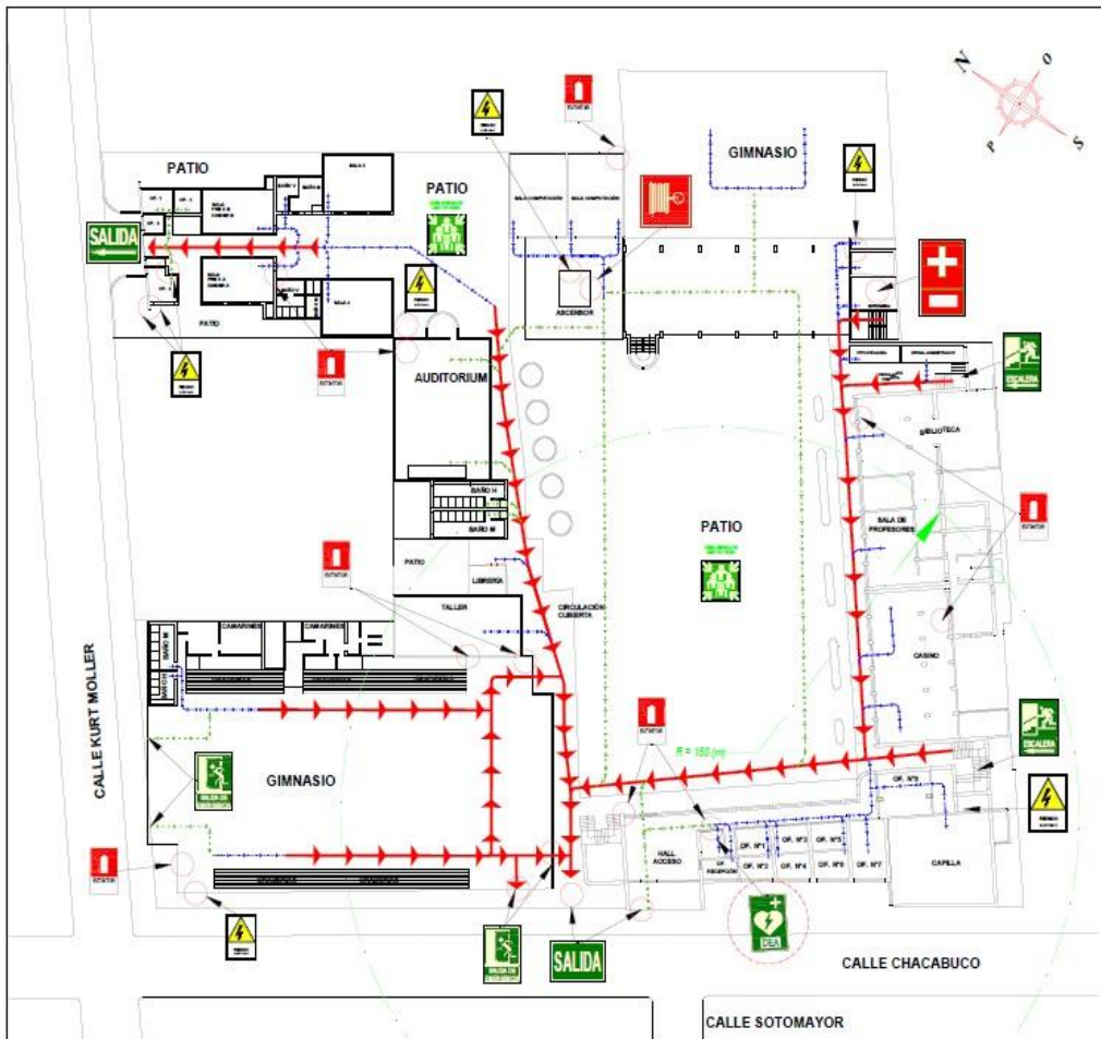
PLANTA 1º NIVEL, INSTITUTO LINARES, PLANO GENERAL DE DISTRIBUCIÓN SEÑALIZACIÓN VÍAS DE EMERGENCIA Y DEA. Esc. 1:250.-
